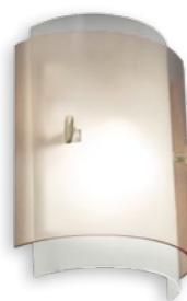
FABAS LUCE Wandleuchte Glas Amber IP20 mit gebogenem Innendiffusor LxBxH: 28,5x23x35,5cm exkl. 1xE27 max. 40W 332 230 34 70,00 €
