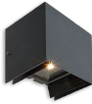
LxBxH: 14x10,5x14,5cm inkl. LED 5,5W 3.000K 200lm
