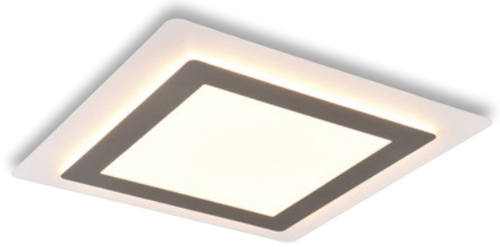
TRIO LED-Deckenleuchte nickel mit Fernbedienung und Nachtlicht LxBxH: 45x45x4,2cm inkl. 1xSMD LED 46W 2.700-6.500K 6.000lm
